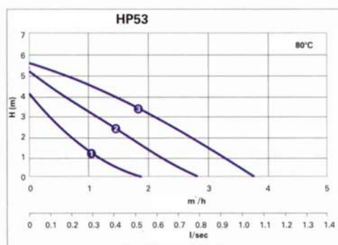
Гидравлические характеристики насоса HP53 (температура воды 80° С, 220 В, 50 Гц.)
